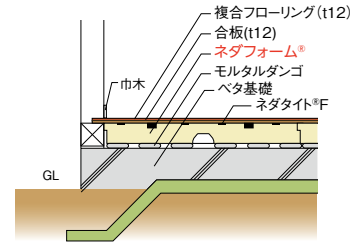
■ベタ基礎
