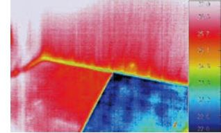
サーモグラフィカメラで撮影した、ネダフォーム®33mm+フローリングとフローリング6mm直貼り床の比較写真 FL表面温度 NFあり:24°C(赤部分) NFなし:18°C(青部分) AC24°C設定、風=上向き
