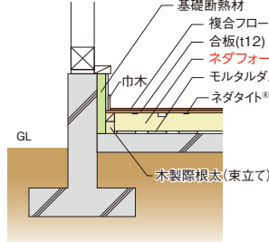
■土間コンクリート(布基礎)
