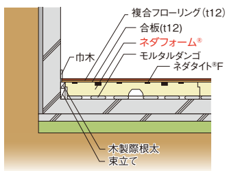
■地下室
