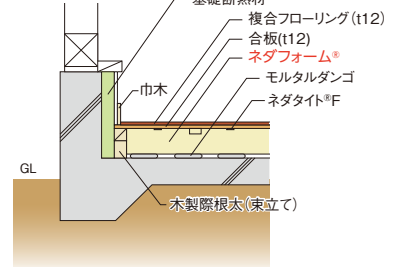
■ベタ基礎
