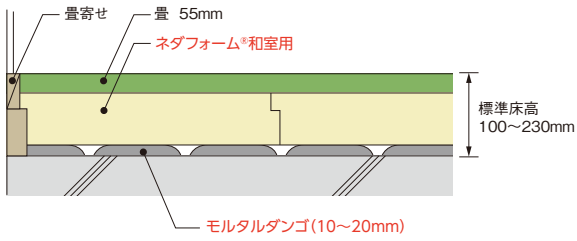
■施工例:ネダフォーム® 和室用 標準的な納まり、壁との取り合い(和室)
