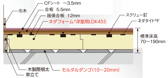
■床暖房(ガス・電気)システムを取り入れる納まり
